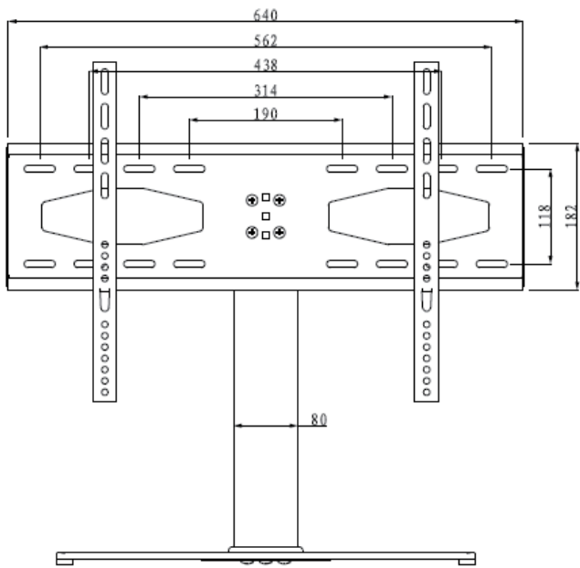
HVDM-SB55 立式支架尺寸图
