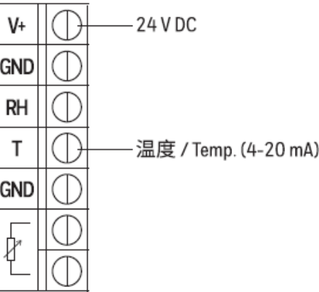
接线图2
