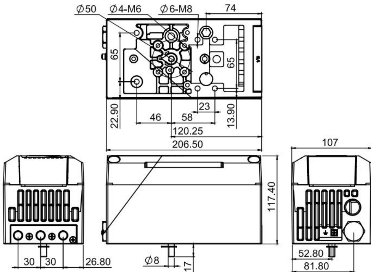
图6 SVP智能阀门定位器外形尺寸图
