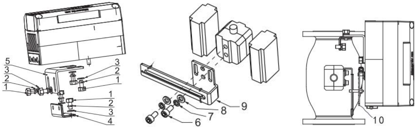
图10 直行程阀门定位器安装连接图
