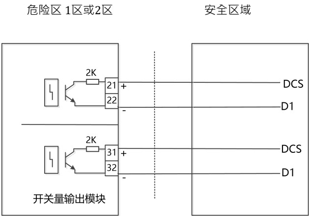
图3 开关量输出模块电气连接图
