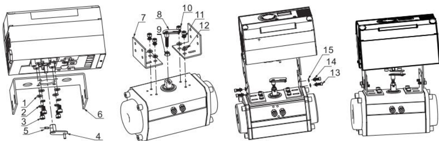
尺寸图：(角行程安装)
