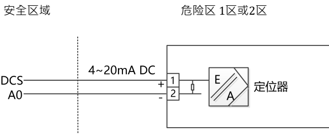
图2 输入电气连接图
