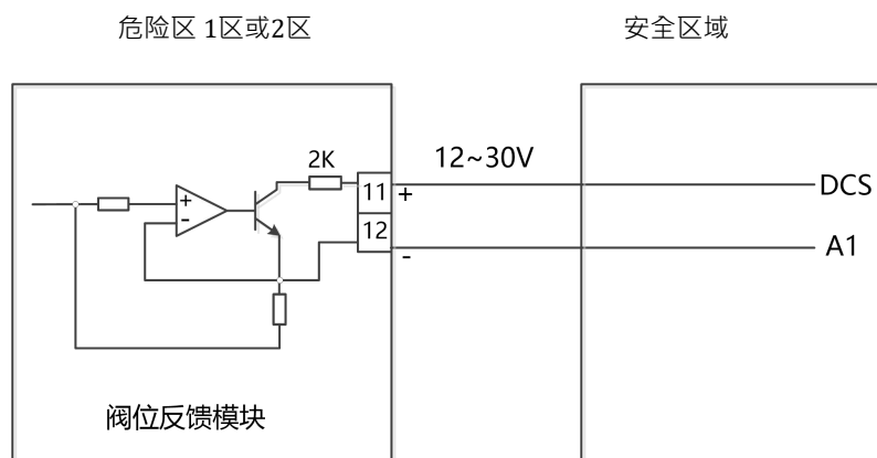
图4 阀位反馈模块电气连接图
