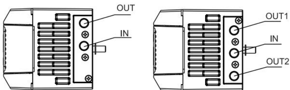
图12 气路连接图
