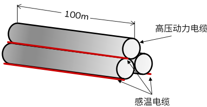
直线敷设式高压电缆安装示意
