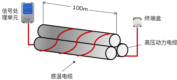
直线敷设式高压电缆安装示意
