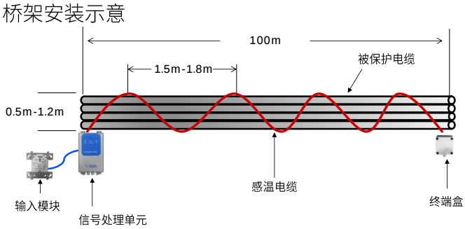
缠绕式高压电缆安装示意
