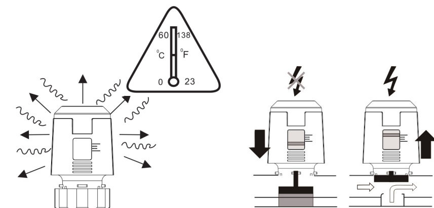
安装示意图
