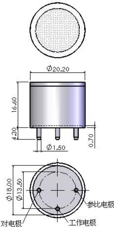
外形尺寸
