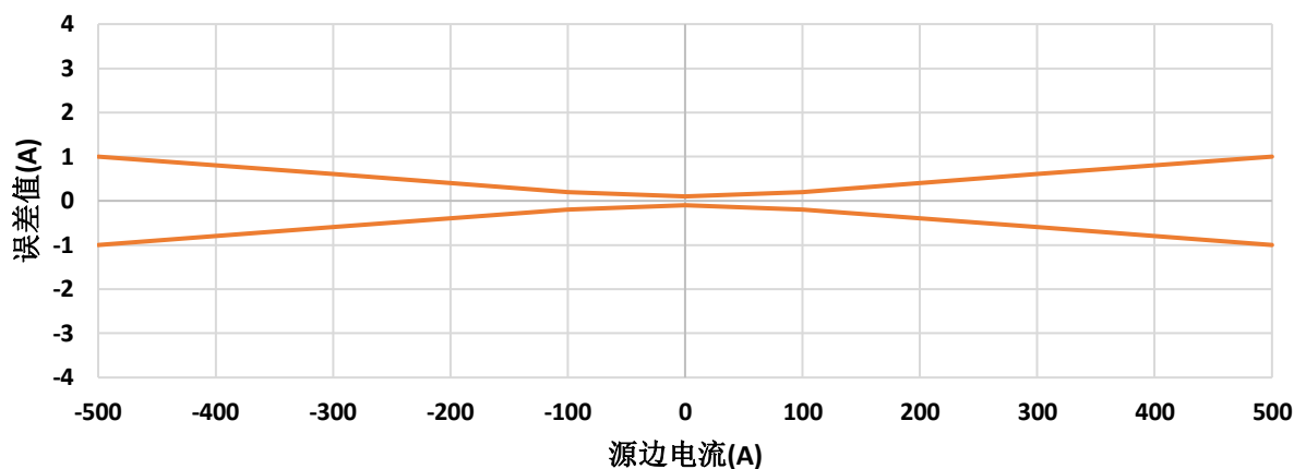
全温精度误差@(-40°C~85°C), \pm 3 Sigma
