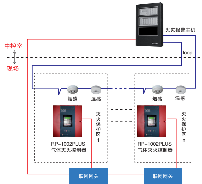
典型多个气灭盘系统图
