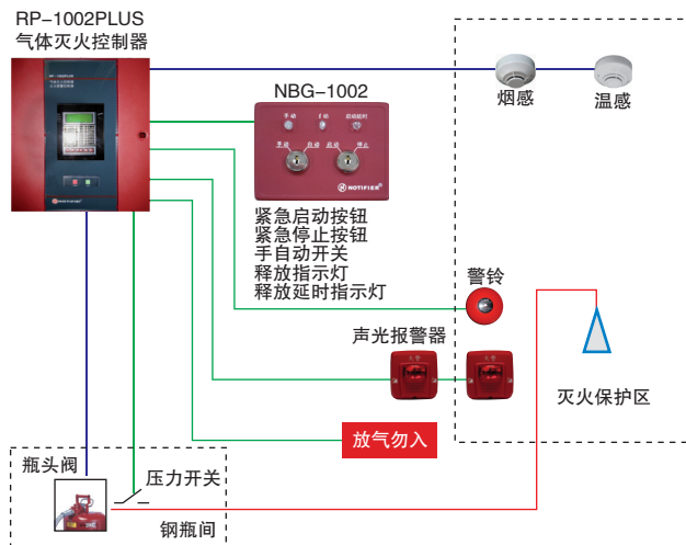
单区气灭盘系统图
