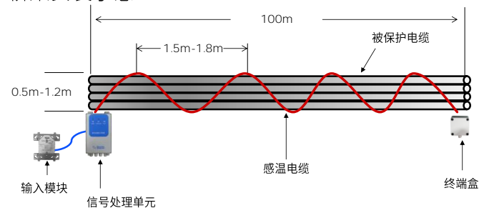
缠绕式高压电缆安装示意
