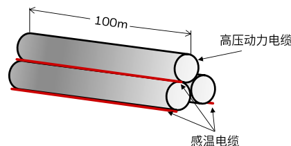
直线敷设式高压电缆安装示意
